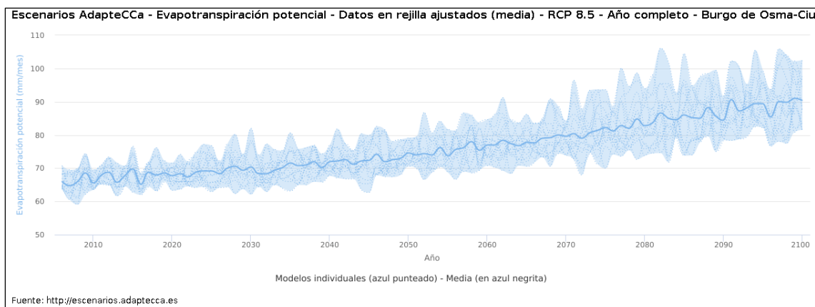
Figura 4: Gráfico de la evolución prevista a lo largo del siglo XXI de la evapotranspiración potencial media en Burgo de Osma. Fuente: Visor de Escenarios de Cambio Climático (adaptecca.es)
