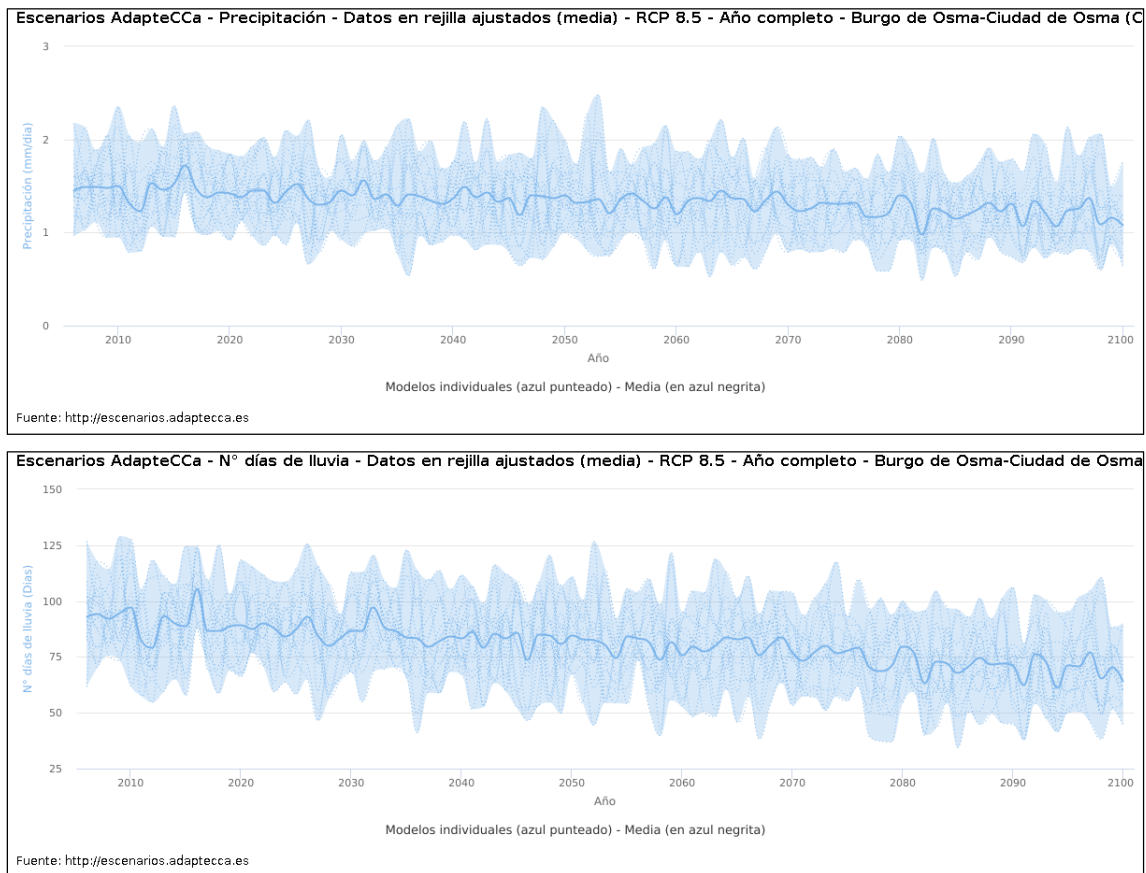
Figura 3: Gráfico de la evolución prevista a lo largo del siglo XXI de la precipitación media y del número medio de días de lluvia en Burgo de Osma. Fuente: Visor de Escenarios de Cambio Climático (adaptecca.es)
