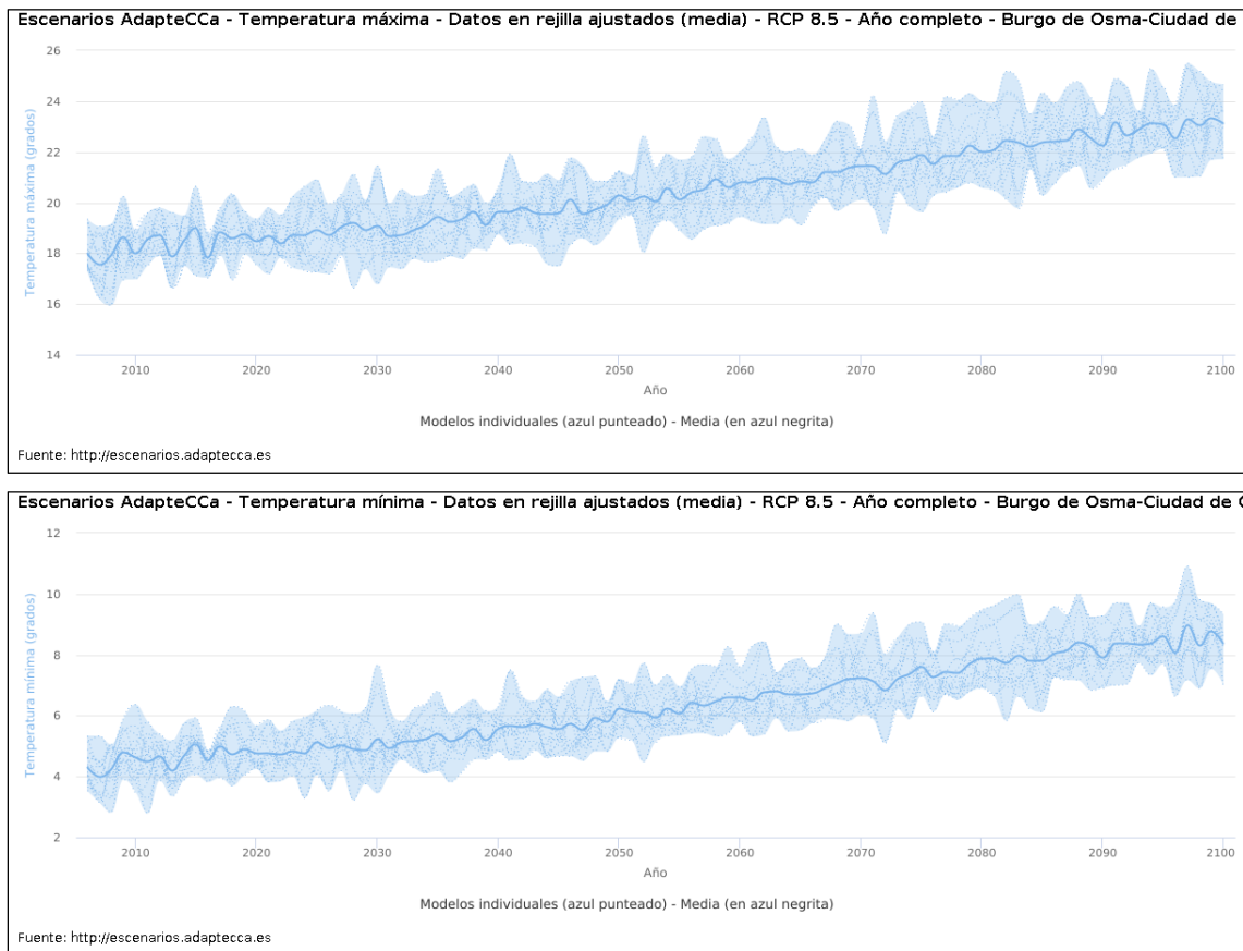
Figura 2: Gráficos de la evolución prevista a lo largo del siglo XXI de las temperaturas máximas medias y de las temperaturas mínimas medias para Burgo de Osma. Fuente: Visor de Escenarios de Cambio Climático ( adaptecca.es )
